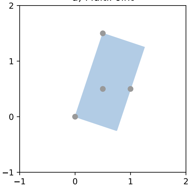
a) MultiPoint
