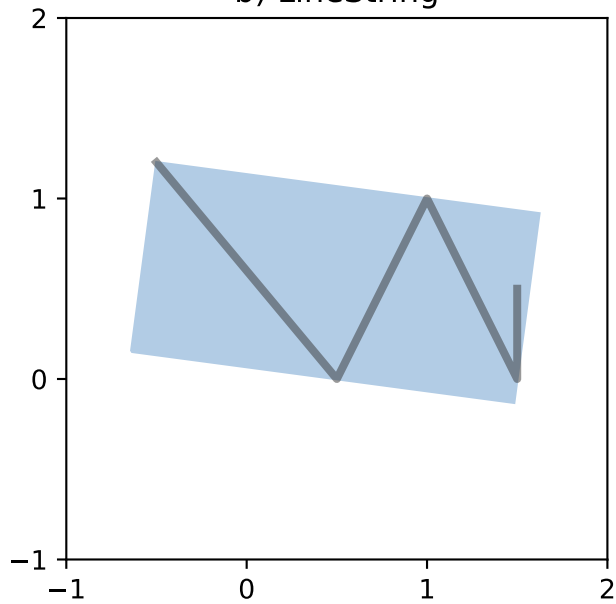
b) LineString
