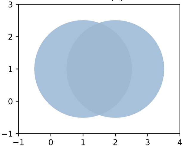
a.union(b)
