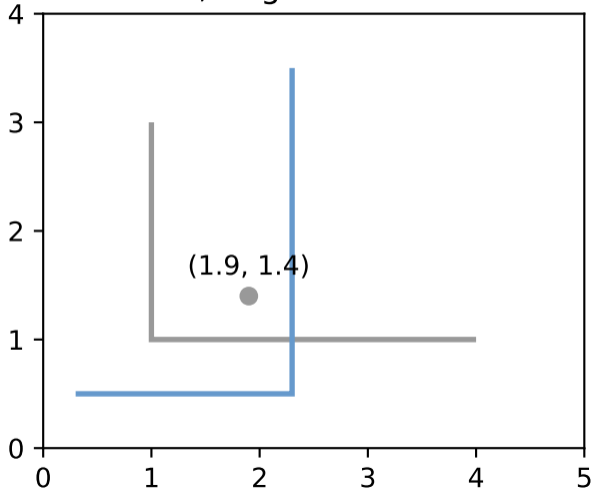
90°, origin='centroid'
