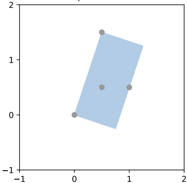
a) MultiPoint
