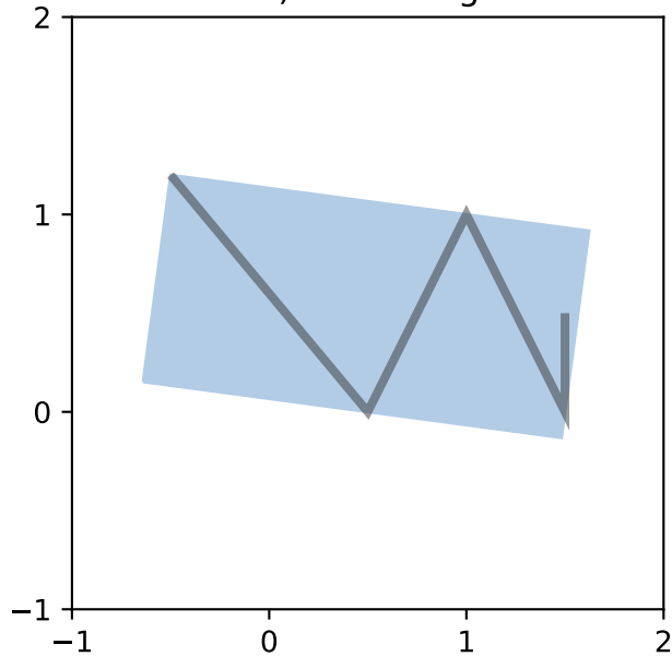
b) LineString
