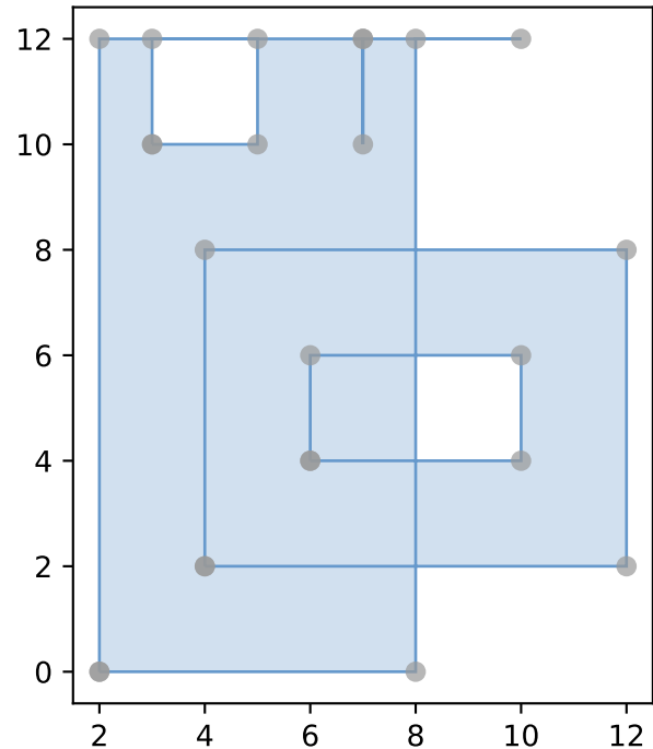
invalid input
